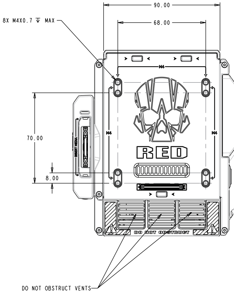
Figure: WEAPON con sensor MONSTRO 8K VV Vista Posterior
