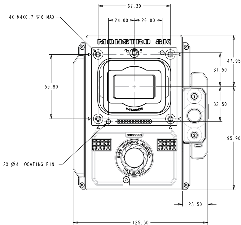
Figure: WEAPON con sensor MONSTRO 8K VV Vista Frontal
