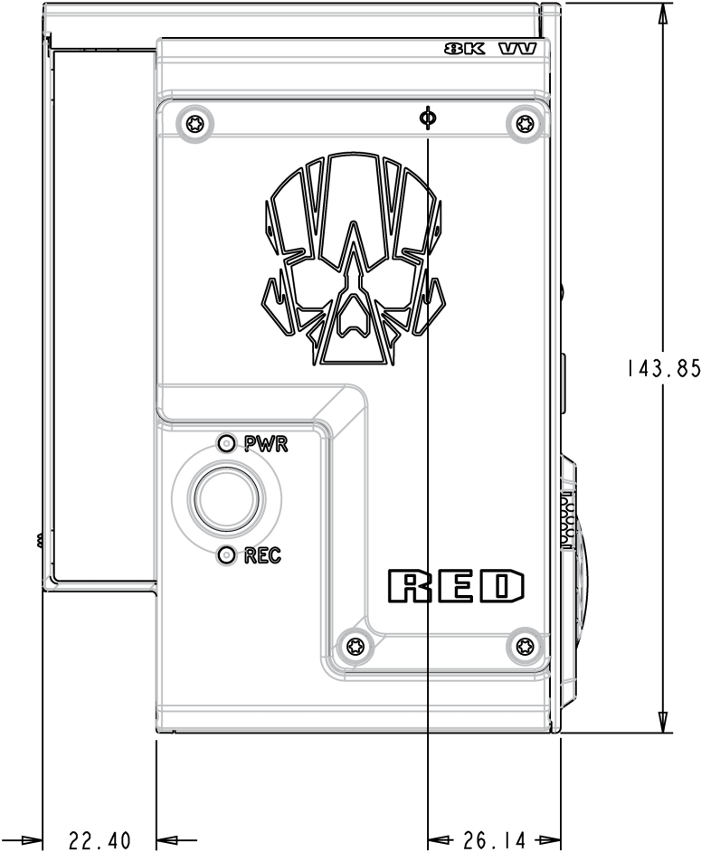
Figure: WEAPON con sensor MONSTRO 8K VV Vista Lateral (Izquierda)
