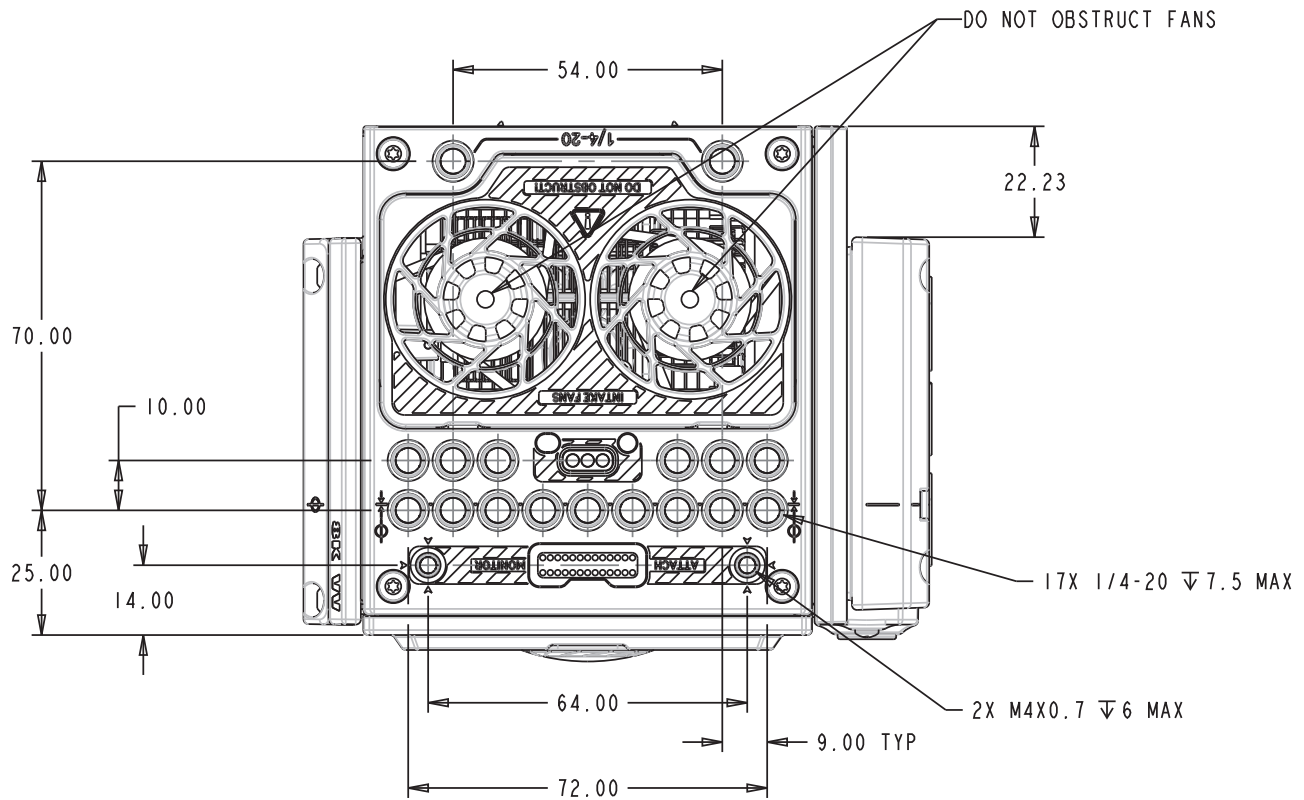
Figure: WEAPON con sensor MONSTRO 8K VV Vista Superior
