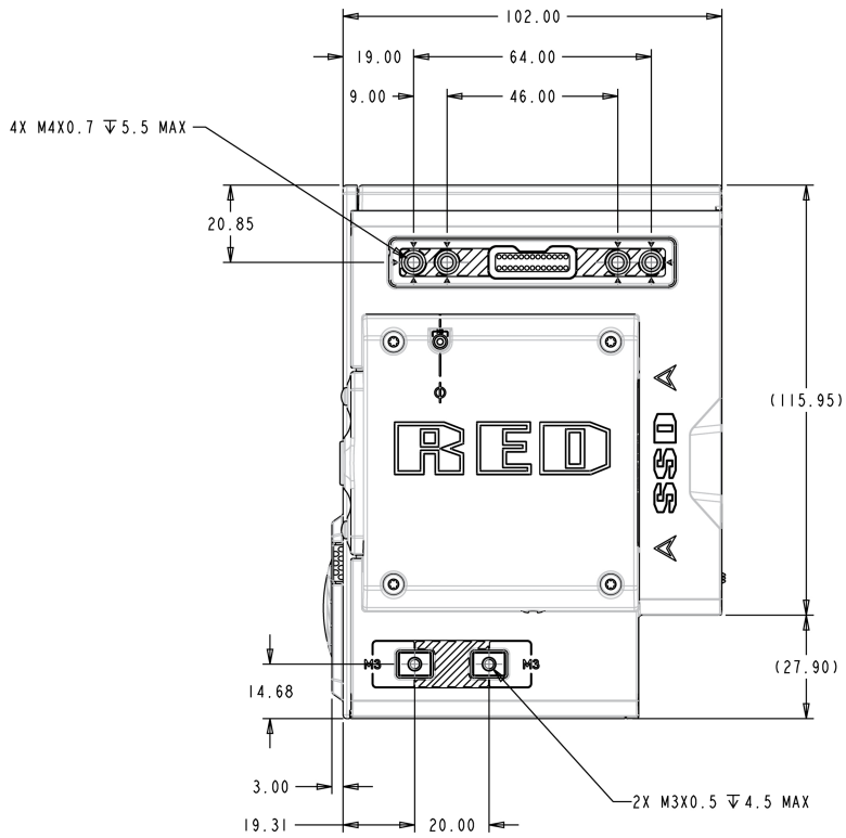
Figure: WEAPON con sensor MONSTRO 8K WV Vista Lateral (Derecha)
