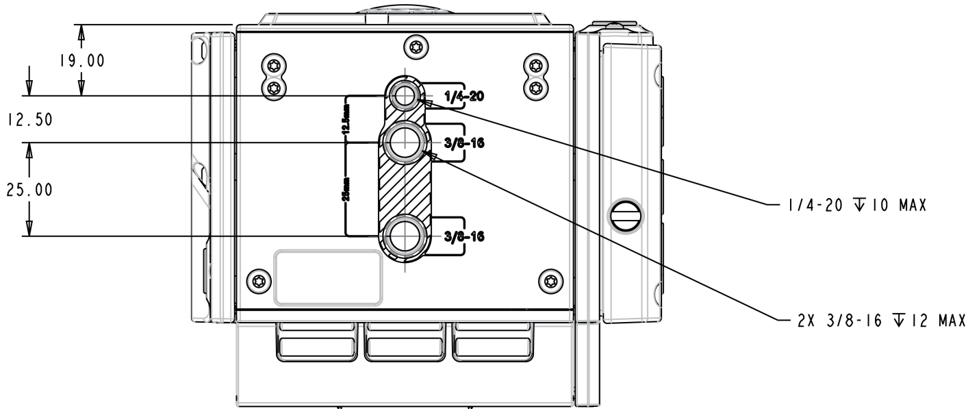
Figure: WEAPON con sensor MONSTRO 8K VV Vista Inferior
